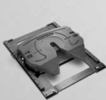
H7 AWB Sistema Deslizable 62,500 lbs carga vertical 150,000 lbs de arrastre
